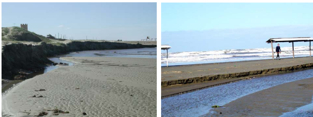
Figura 2.8 – Erosão causada por sangradouro. (Foto: autor)
