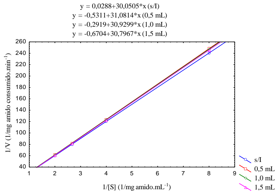
Figura 11 - Gráfico de duplo-recíproco de Lineweaver-Burk para o feijão carioca amendoim.
