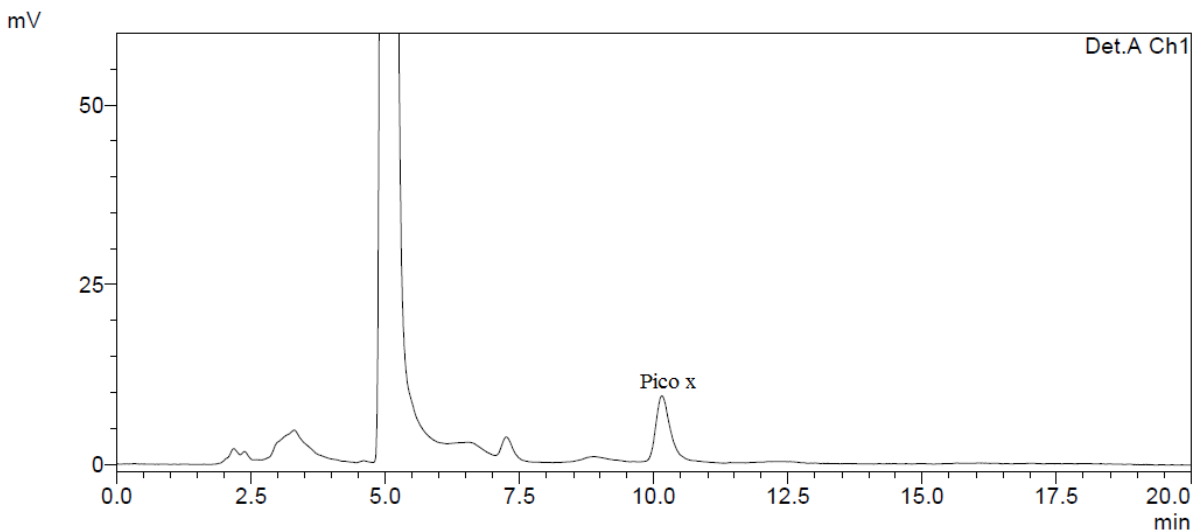
Figura 8 - Cromatograma de eluição do extrato de AFLAs do feijão vermelho obtidos através de HPLC-FL.
