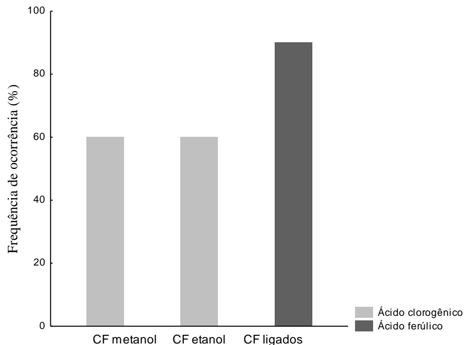
Figura 3 - Percentual de frequência de ácidos fenólicos predominantes nas variedades de feijões.
