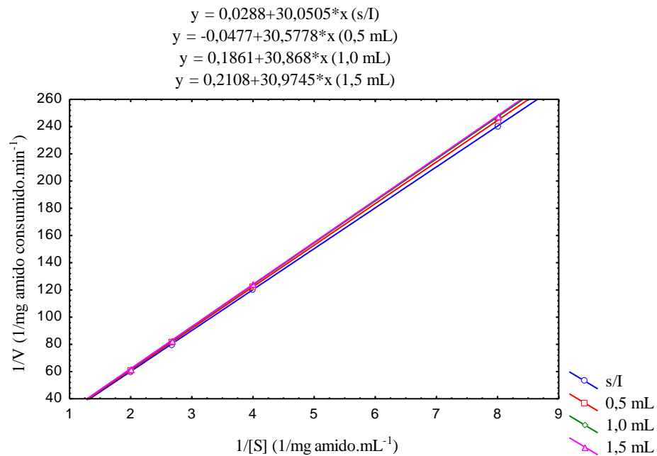
Figura 10 - Gráfico de duplo-recíproco de Lineweaver-Burk para o feijão carioca azuki.
