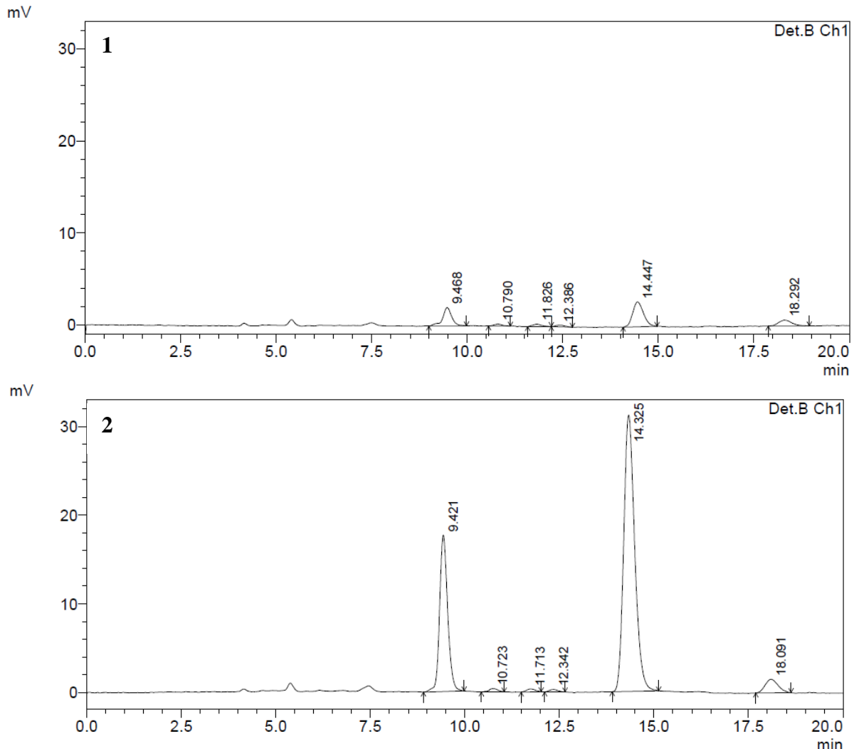
Figura 6 – Cromatogramas das AFLAs B 1 , B 2 , G 1 e G 2 obtidos através de HPLC-FL. Sendo 1 : Segundo ponto da curva (concentrações de 8,0 ng.mL -1 para as AFLAs B 1 e G 1 e 0,5 ng.mL -1 para as AFLAs B 2 e G 2 ) ; 2 : quinto ponto da curva (concentrações de 15,0 ng.mL -1 para as AFLAs B 1 e G 1 e 5 ng.mL -1 para as AFLAs B 2 e G 2 ).
