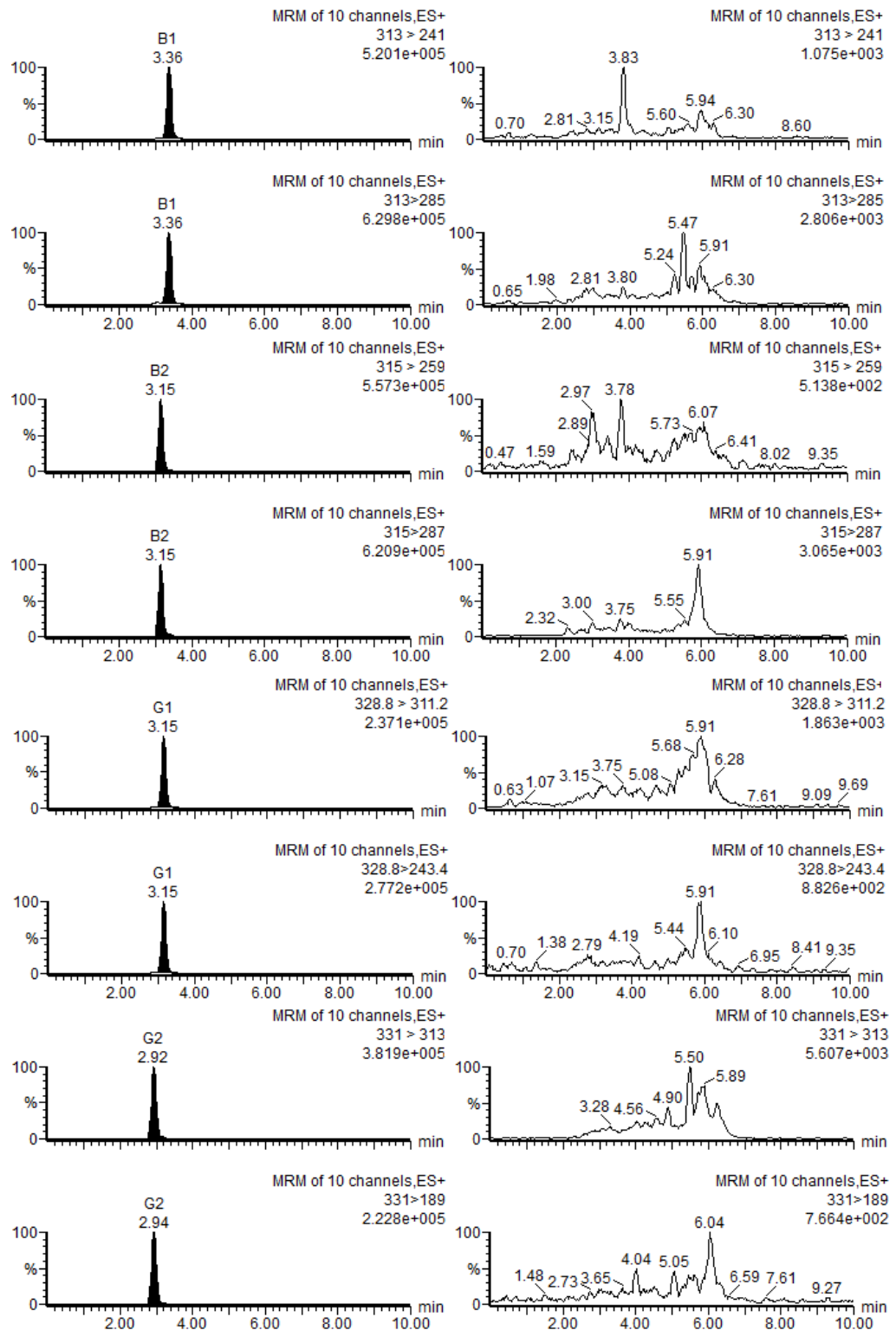
Figura 9 – Cromatogramas de eluição dos padrões de AFLAs e do extrato de AFLAs do feijão vermelho em LC-ESI-MS/MS. Onde: Lado esquerdo representa os padrões de AFLAS ( 1 \text{ mg.L}^{-1} ) e as duas transições de cada composto; Lado direito representa o extrato da amostra.
