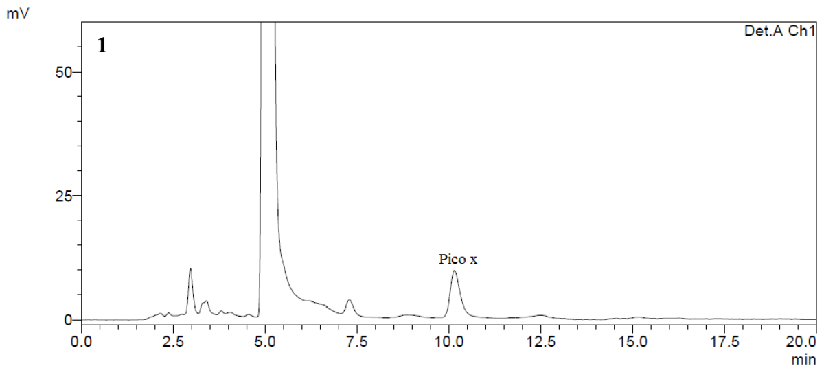
Figura 7 - Cromatogramas de eluição do extrato de aflatoxinas obtidos através de HPLC-FL.
