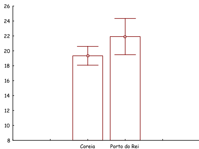
Figura 13 - Valores médios e erro padrão da salinidade ao longo do ciclo de produção na localidade da Coreia e do Porto do Rei, Ilha dos Marinheiros, Rio Grande, RS.
