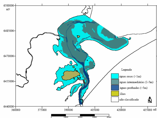
Figura 10 – Mapa com as principais isóbatas presentes nas cartas batimétricas (Fonte: Freitas 2003).
