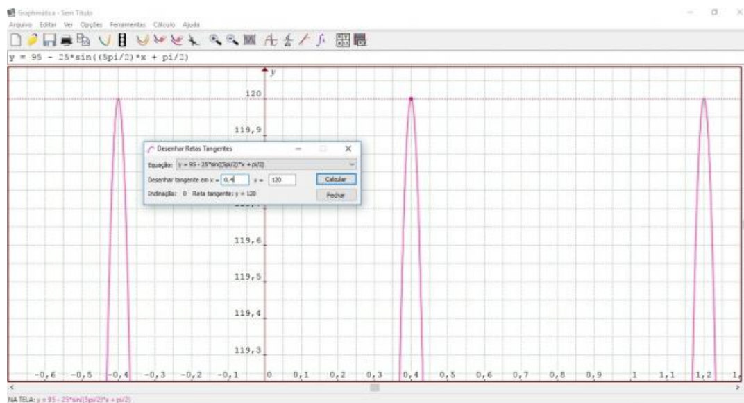
Figura 77 – Gráfico da função y = 95 - 25 \sin\left(\frac{5\pi}{2}x + \frac{\pi}{2}\right) com tangente no ponto (4/10, 120) .
