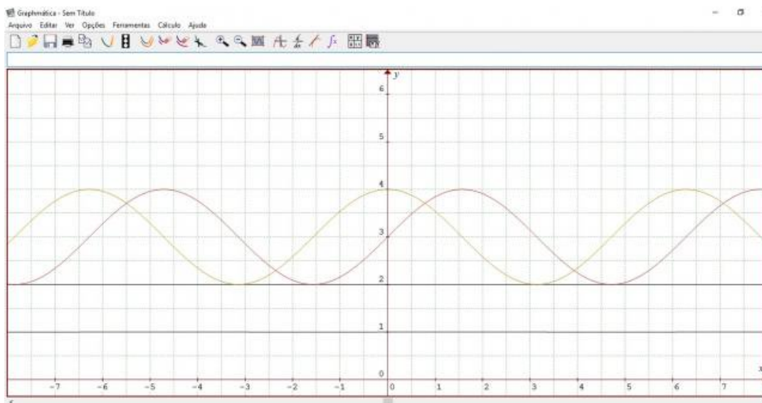
Figura 57 – Gráfico das funções y = 3 + \sin(x)\{x : -8, 8\} e y = 3 + \cos(x)\{x : -8, 8\} .
