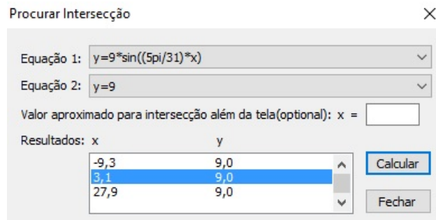
Figura 70 – Intersecções das funções y = 9 e y = 9 * \sin(\frac{5\pi}{31}x) .
