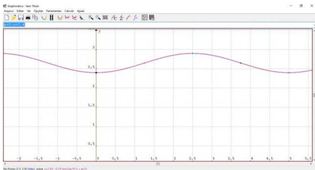
Figura 73 – Pontos sobre o gráfico da função y = 2,65 - 0,25 \sin\left(\frac{2\pi}{5}x + \pi/2\right) .
