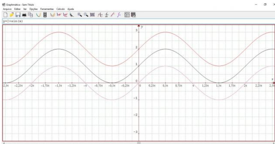
Figura 45 – Solução do gráfico y = a + \text{sen}(x) .
