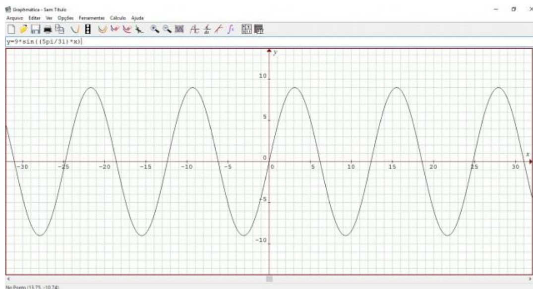
Figura 66 – Gráfico da Função y = 9 * \sin(\frac{5\pi}{31}x) .
