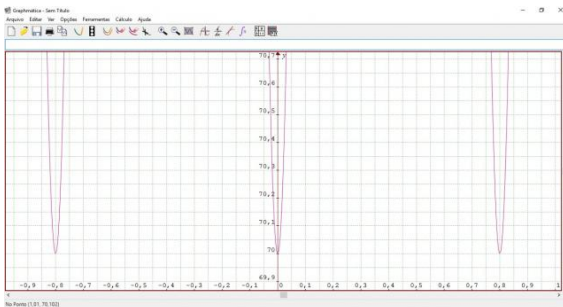
Figura 78 – Observação 1 do gráfico da função y = 95 - 25 \sin\left(\frac{5\pi}{2}x + \frac{\pi}{2}\right) .
