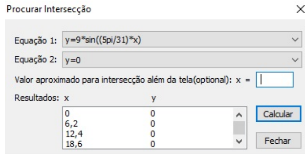
Figura 69 – Intersecções das funções y = 0 e y = 9 * \sin(\frac{5\pi}{31}x) .
