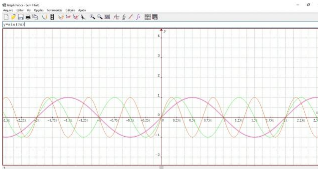
Figura 47 – Solução do gráfico y = \text{sen}(c \cdot x) .
