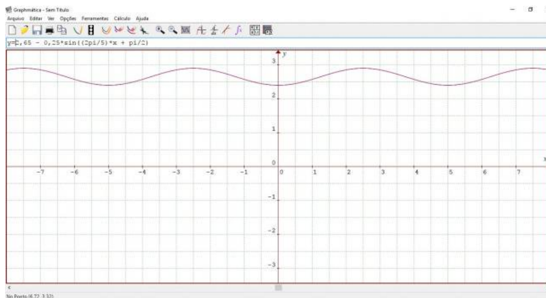
Figura 72 – Gráfico da função y = 2,65 - 0,25 \sin\left(\frac{2\pi}{5}x + \pi/2\right) .
