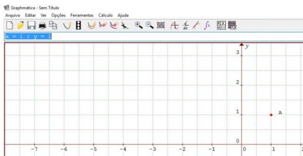
Figura 34 – Ponto A (1, 1).
