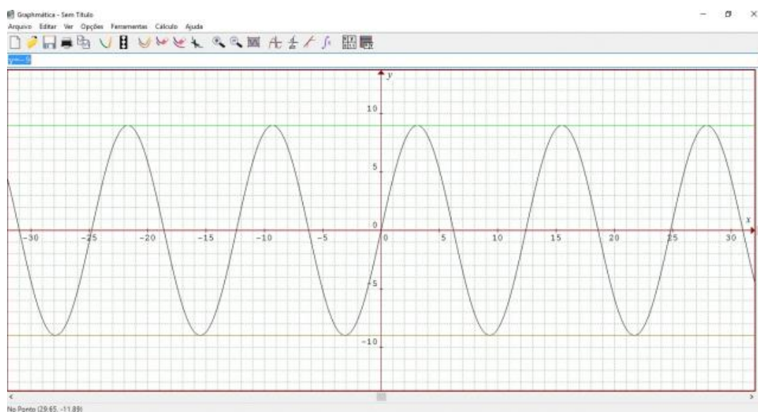
Figura 67 – Gráfico da Função y = 9 * \sin(\frac{5\pi}{31}x) , y = 9 , y = 0 , y = -9 .
