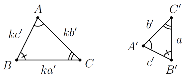
Figura 7 – Dois triângulos semelhantes.
