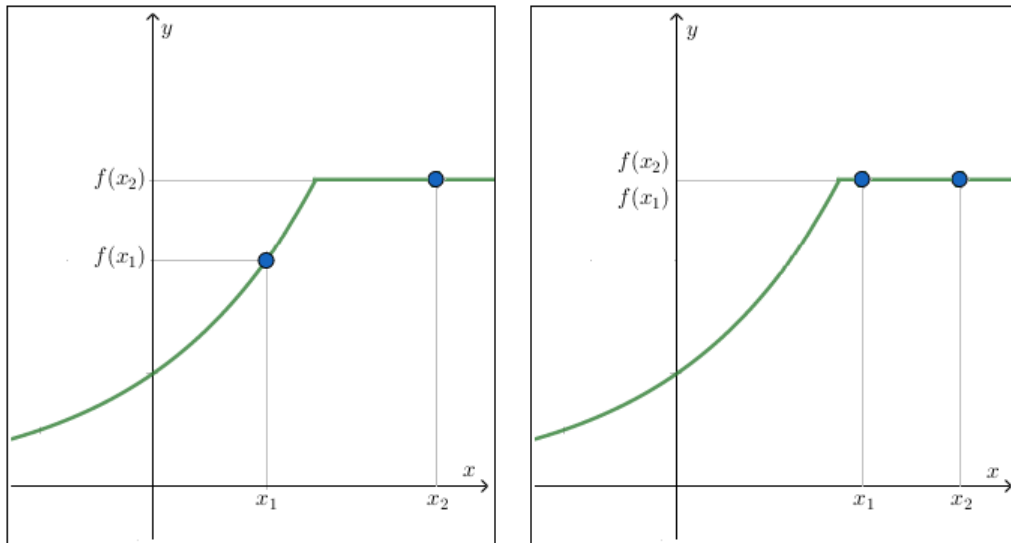
Figura 3 – Representação gráfica de uma função não decrescente.
