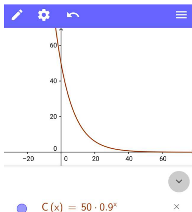
Figura 28 – Gráfico da função C(x) = 50 \cdot (0,9)^x .
