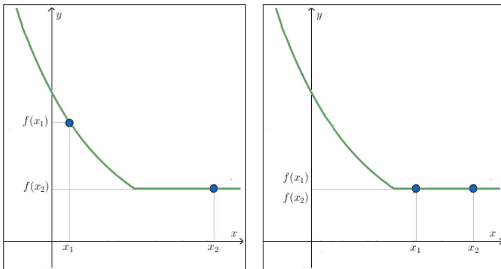
Figura 4 – Representação gráfica de uma função não crescente.
